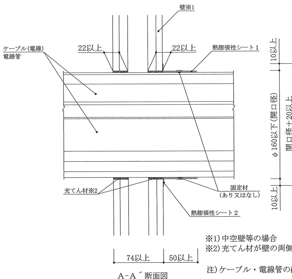
図1 構造説明図
