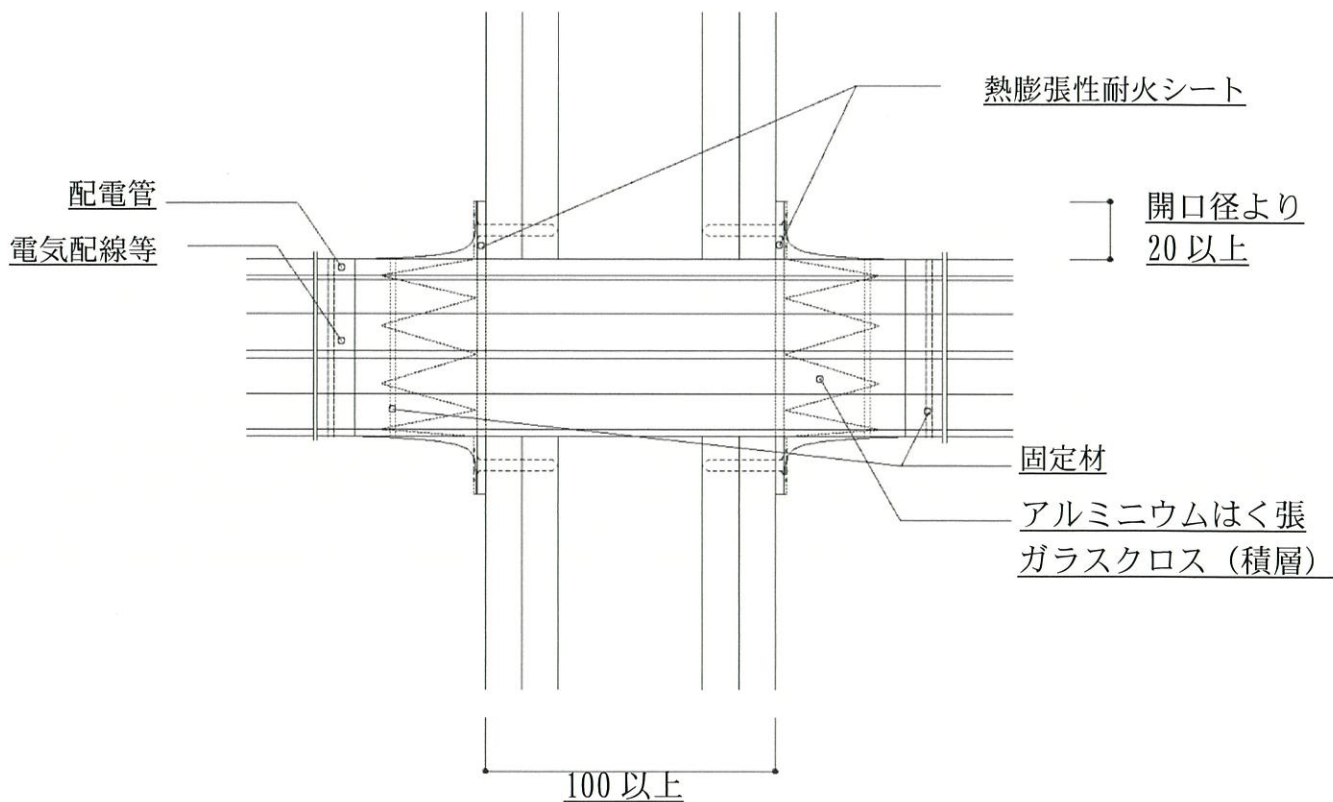
< 断面図 >
