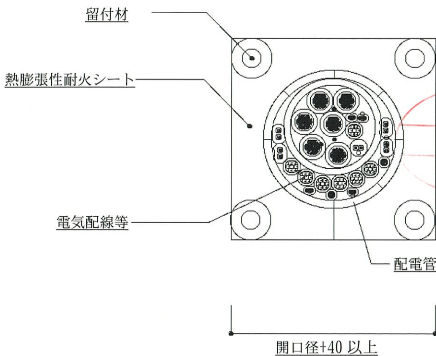
< 正面図 >
