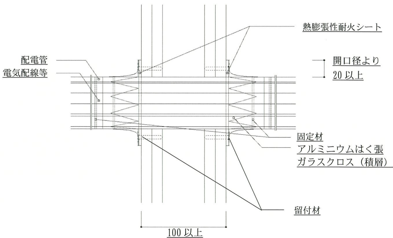
< 断面図 >
