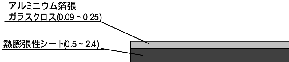
図 - 1 熱膨張性耐火シートの構造
